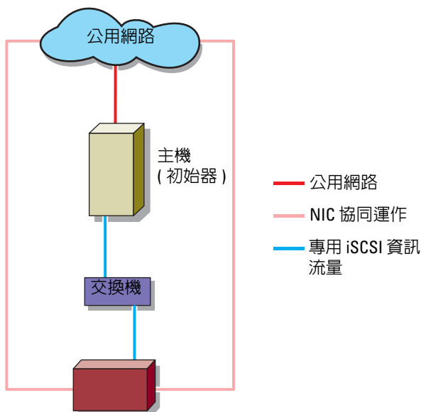
用於資料共用的帶有 NIC 協同運作的 PowerVault NX1950 儲存解決方案
