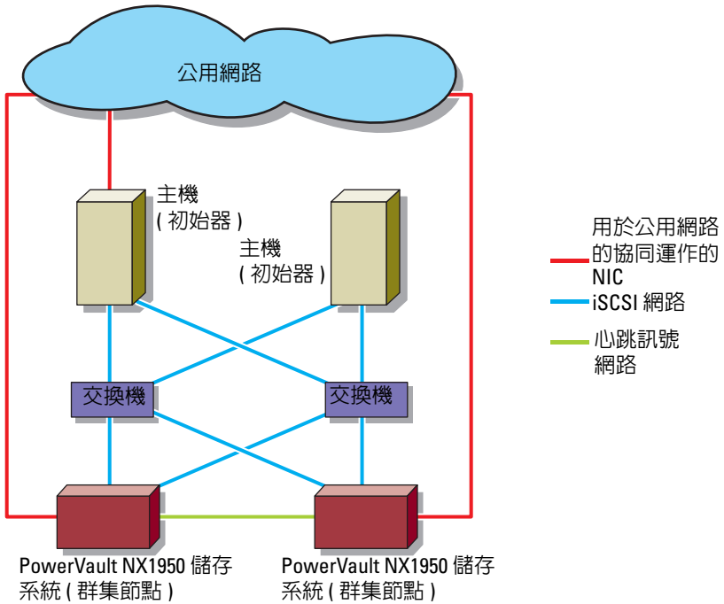
圖 1-4. 使用四個 NIC 的冗餘 iSCSI 路徑
